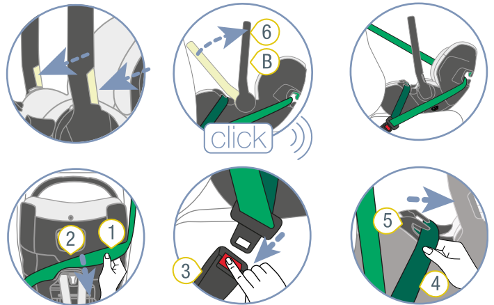
1 Diagonalgurt 2 Gurthalterung 3 Fahrzeuggurtschloss 4 Beckengurt 5 Gurtführungen 6 Tragebügel
